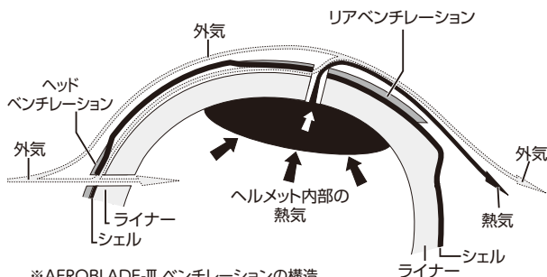
※AEROBLADE-III ベンチレーションの構造
